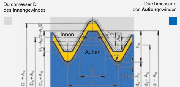
Gewindepassung grob mit weitem Flankenspiel (G/g- oder G/e-Passung) durch Grundabmaß am Außengewinde und im Innengewinde
