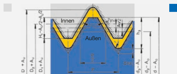
Gewindepassung grob mit weitem Flankenspiel (G/g- oder G/e-Passung) durch Grundabmaße am Außengewinde und im Innengewinde
