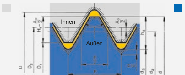
Gewindepassung mittel mit engem Flankenspiel (H/h- oder H/e-Passung) durch Grundabmaß am Außengewinde
