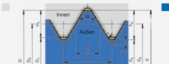
Gewindepassung fein ohne Flankenspiel (H/h-Passung)
